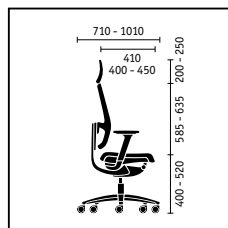
Drehstuhl mit membranbespannter Rückenlehne, 3-D verstellbaren Armlehnen, pulverbeschichtetem Aluminiumfuß in schwarz
